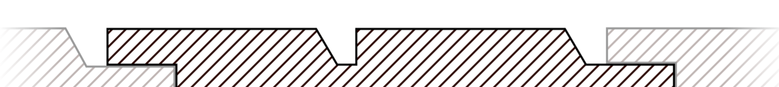
Dobbelfals NS m/spor - 60°
